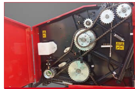
Fácil acceso lateral de la máquina para su mantenimiento. Easy maintenance access.
