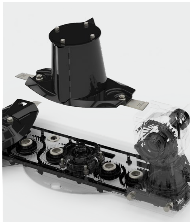
Cono convogliatore per andana stretta (di serie). Disco trasportador para hilera estrecha (estándar).
