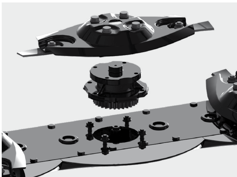
Sezione di sicurezza per la protezione della catena di ingranaggi. Sección de seguridad para la protección de los engranajes.
